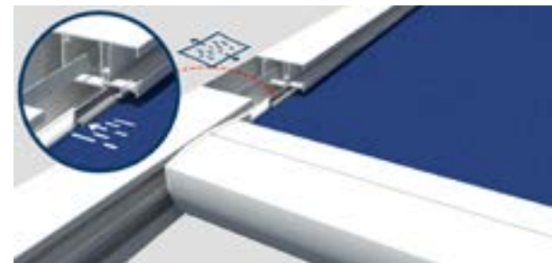
Eine kontinuierlich straffe Tuchspannung dank der ZIP-Screen-Technologie
