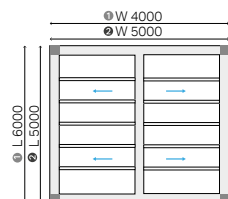
B700 doppeltes Dach
